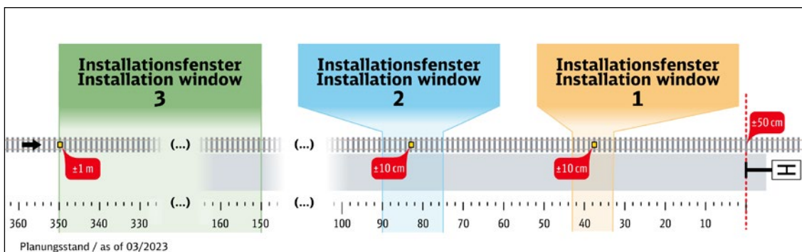
Bild 6: Verlegefenster für „Präzisionshaltbalisen“ Fig. 6: The windows to lay the “precision stop balises”
