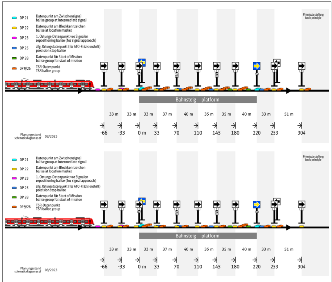
Bild 7: Balisenteppich an einer fiktiven, brettbenen Station vor Optimierung (oben) und mit bisherigen Optimierungen (unten)
