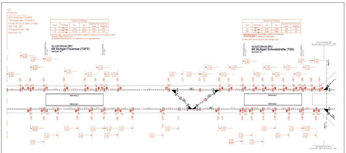
Bild 3: Vereinfachter Auszug aus einem LST-Übersichtsplan der Stammstrecke
